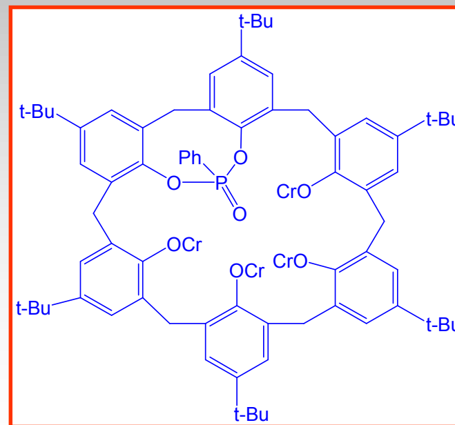
Phenylphosphinoxyde-crotyl p-tert-butyl-calix[6]arene
